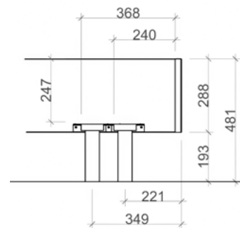
Betttraverse zu 288
