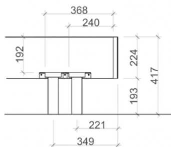
Betttraverse zu 224
