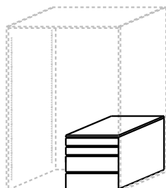
Schubladeninnenkorpus zu Elementbreite 1100 mm
