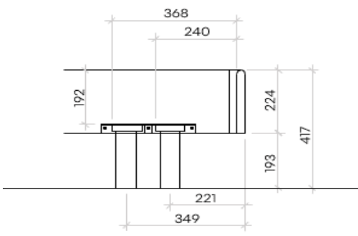
Betttraverse zu 224
