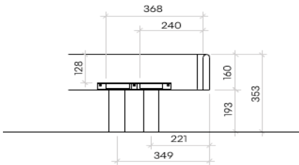
Betttraverse zu 160
